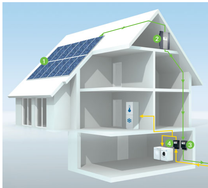
Schemat typowej domowej instalacji fotowoltaicznej
